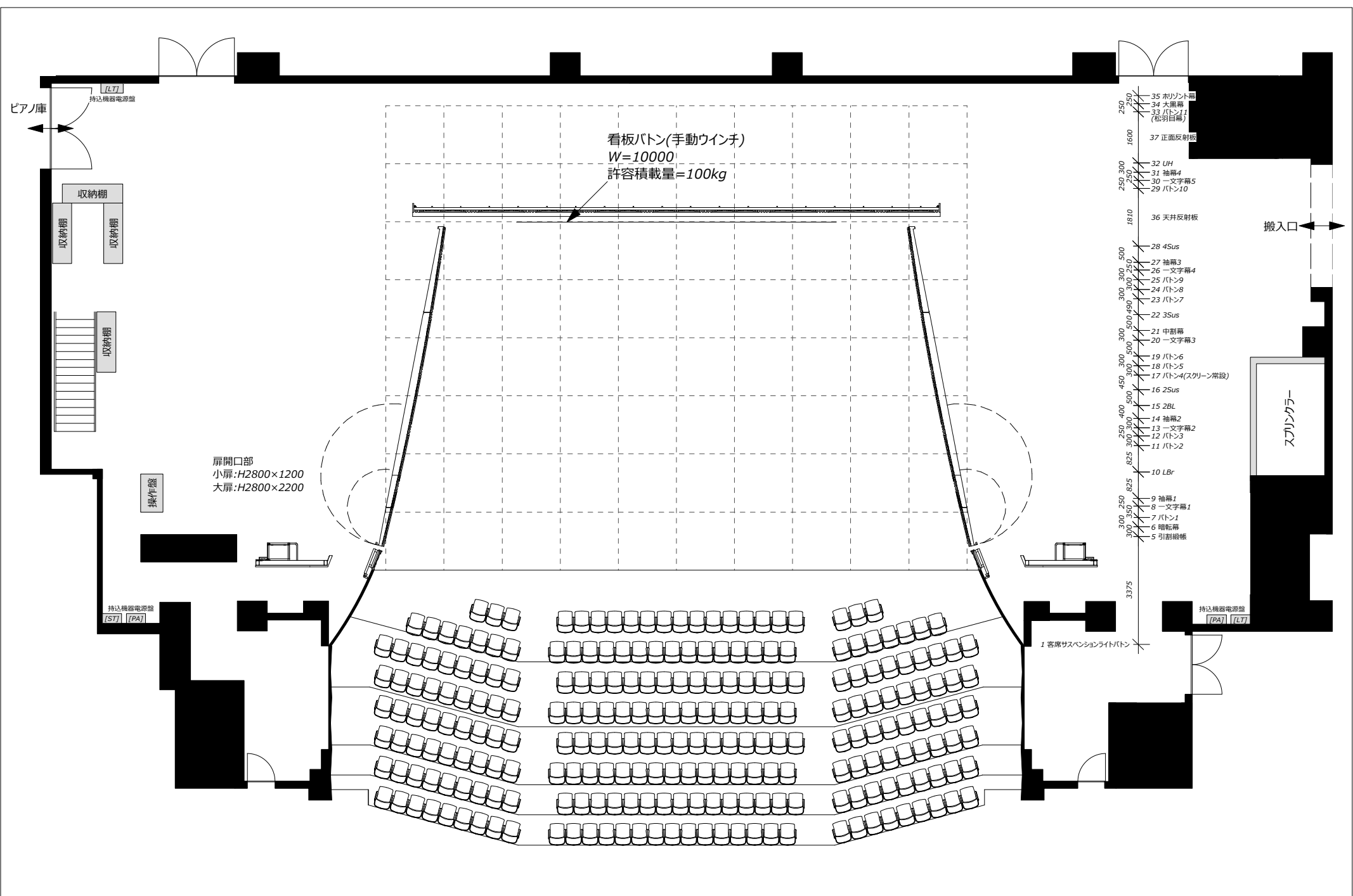
太田市民会館 反響板仕様(大編成) 平面図
