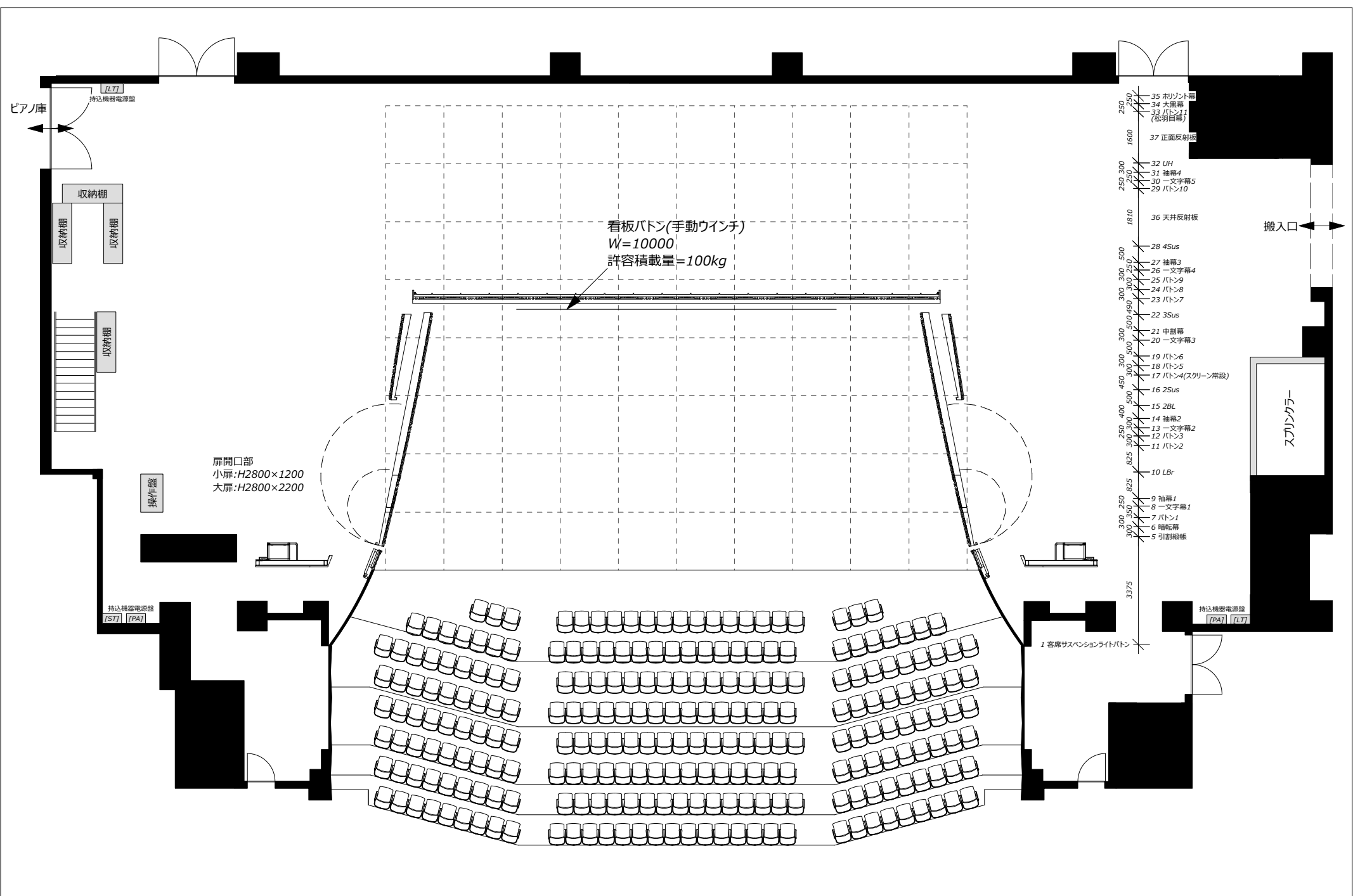
太田市民会館 反響板仕様(中編成) 平面図
